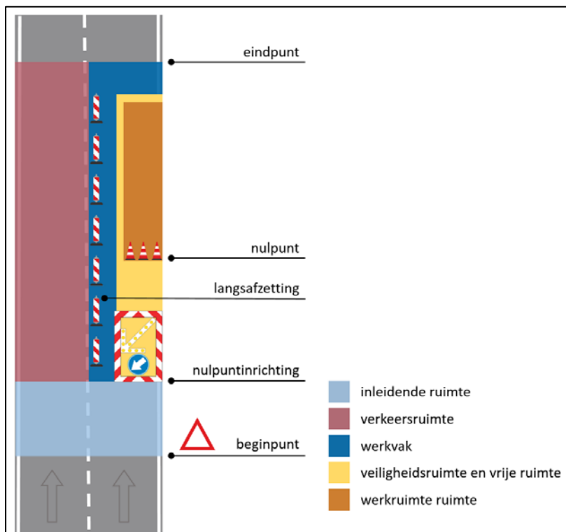
Figuur 2 Overzicht basisopbouw verkeersmaatregelen
